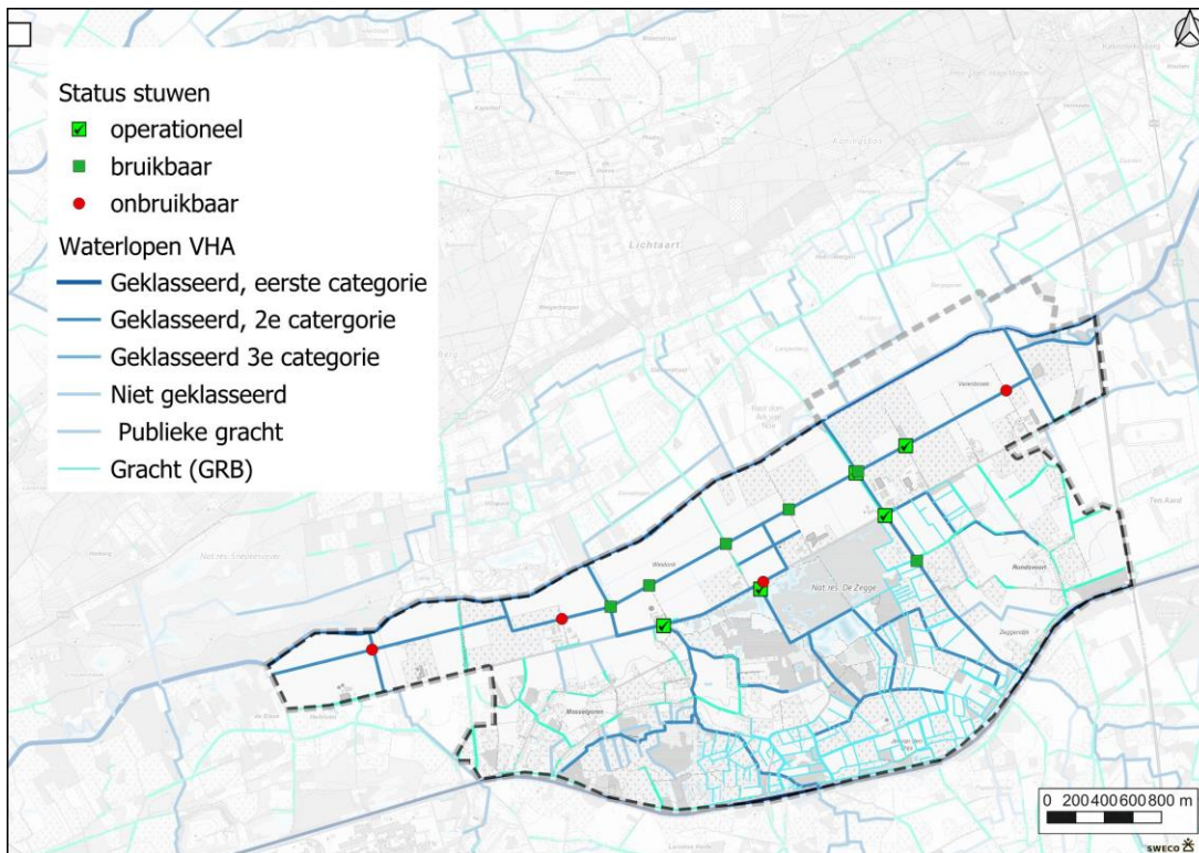
Figuur 20: Status van de stuwen binnen het peilgebied.
