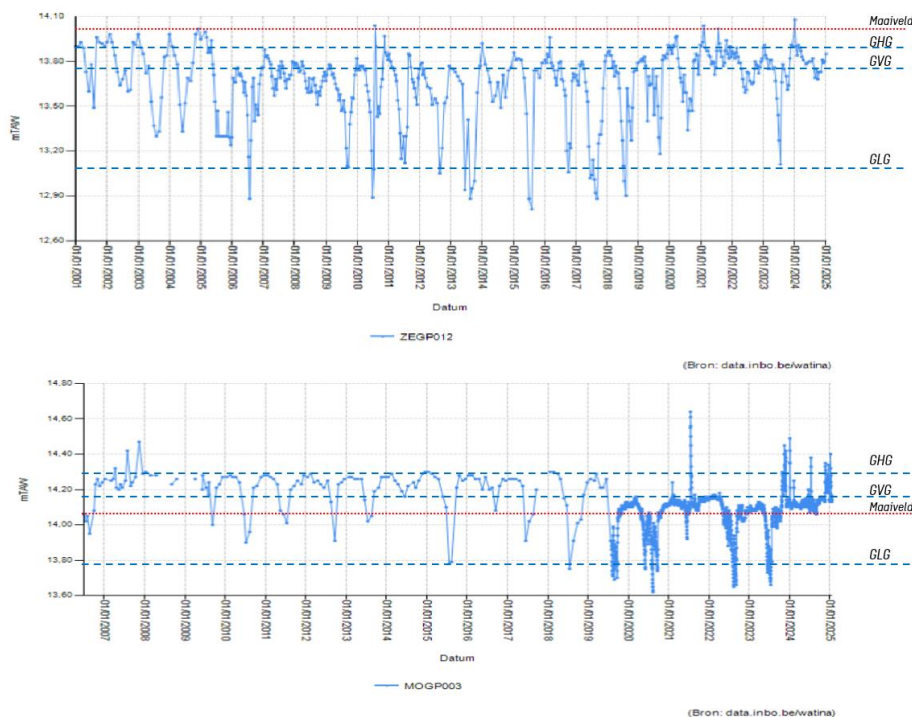
Figuur 27: Meetreeksen van grondwaterstanden die representatief zijn voor De Zegge (boven) en Mosselgoren (onder). (Watina-databank, geraadpleegd op 21 mei 2025).
