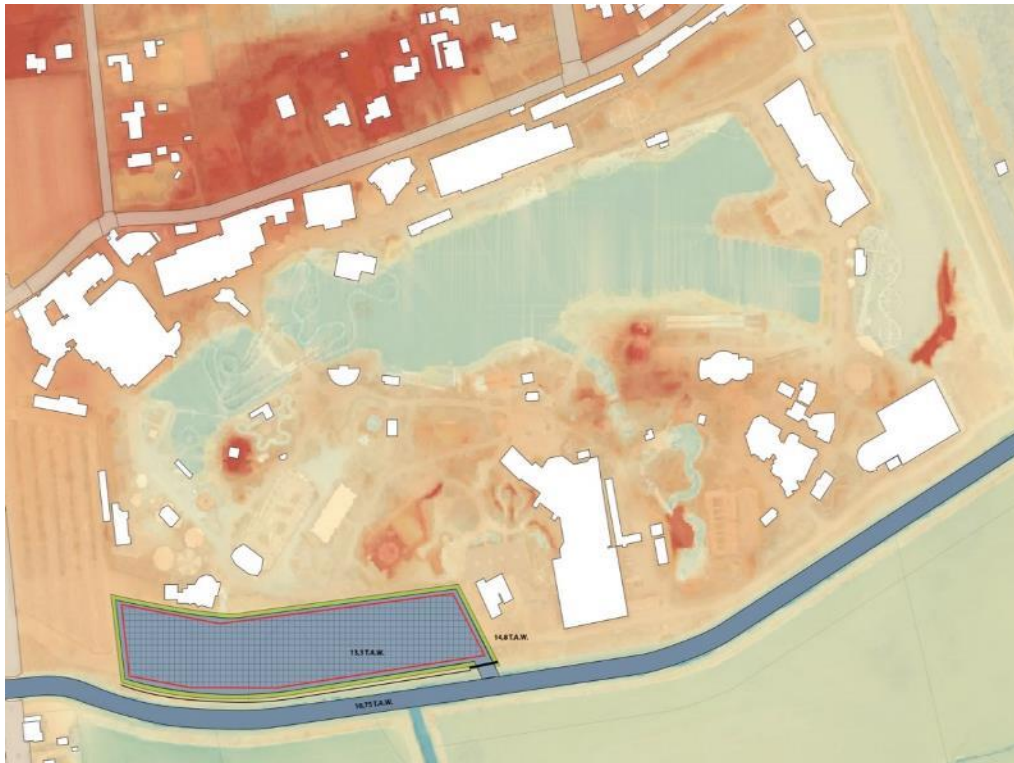
Parking als tijdelijk waterbergingsgebied (dmv inlaatconstructie)
